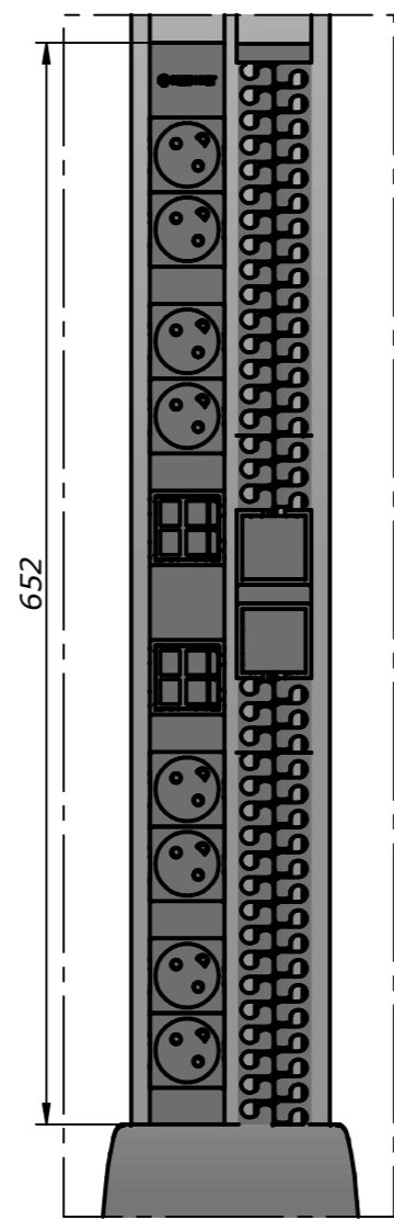
DETALLE A
